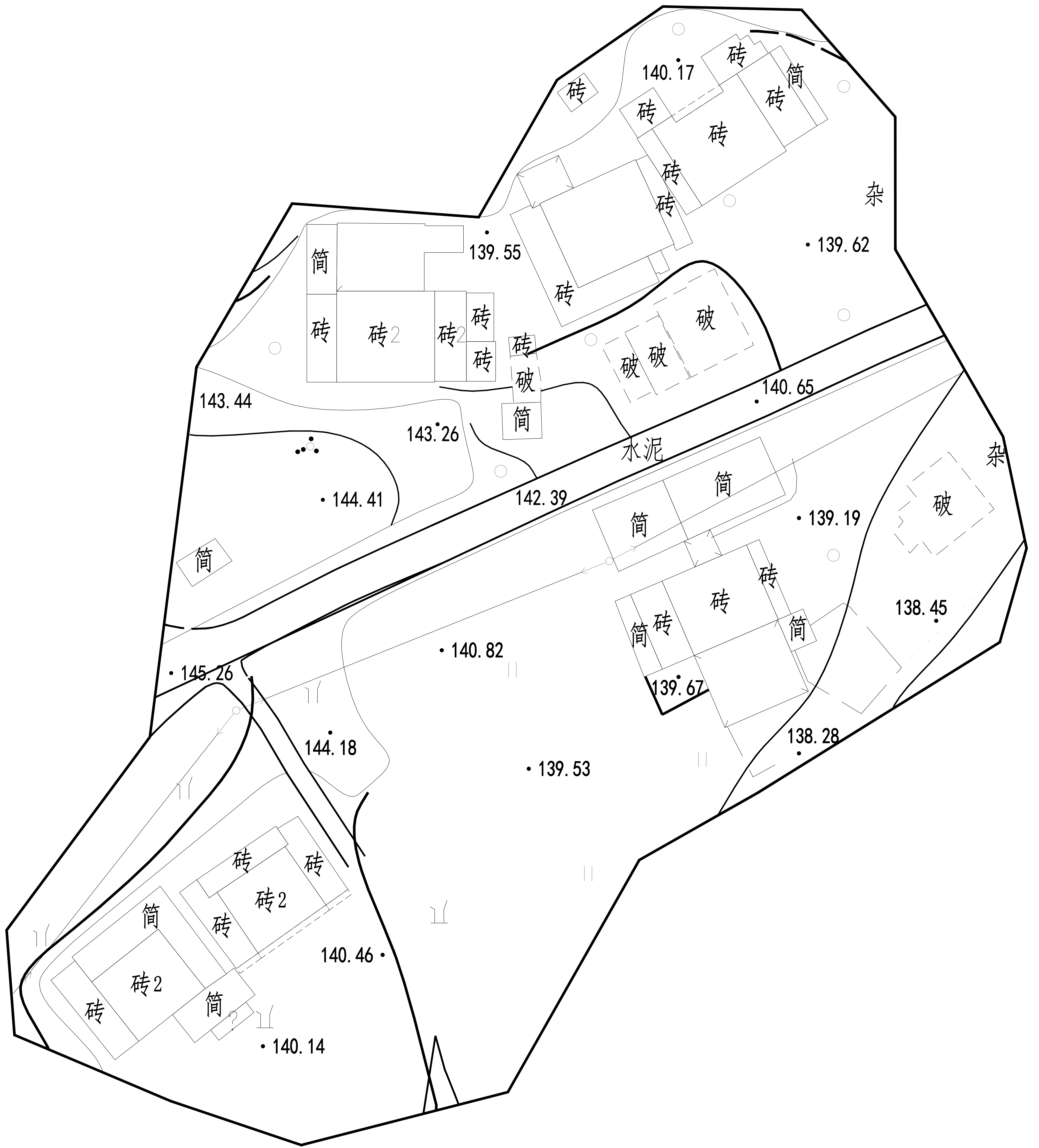
房屋拆除范围内建（构）筑物红线图
